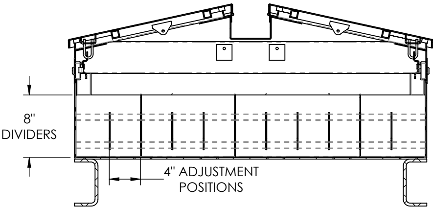
SECTION B-B SCALE 1 : 12
