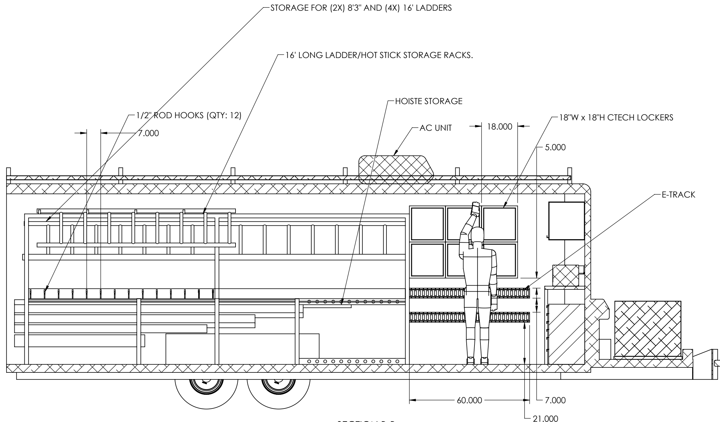
SECTION B-B SCALE 1 : 30
