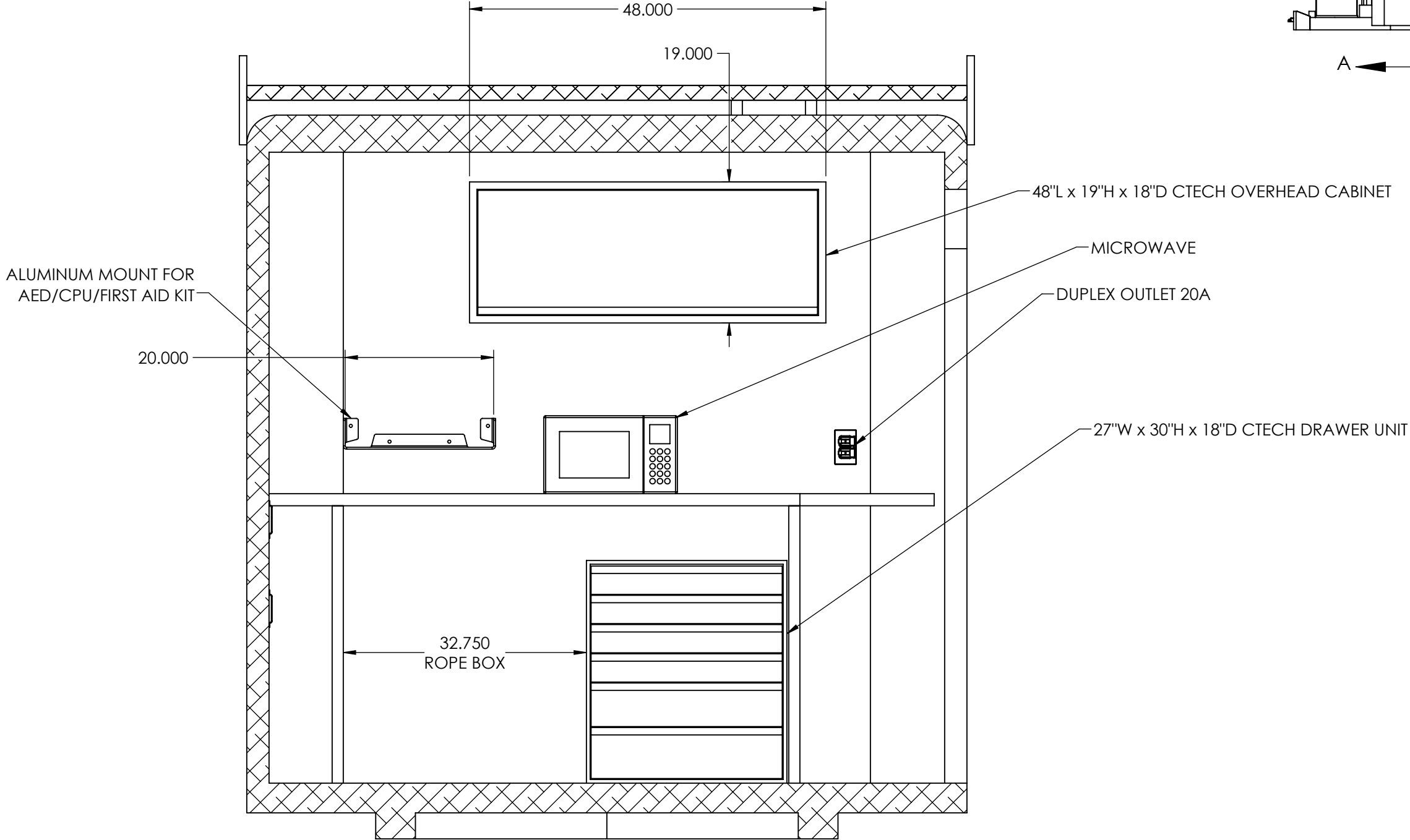
SECTION A-A SCALE 1 : 16
